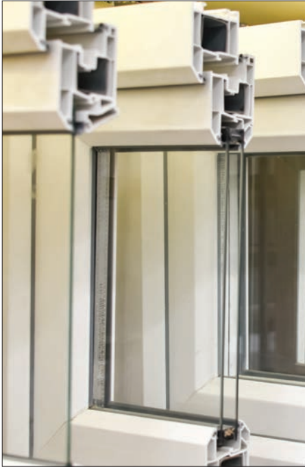
Doble acristalamiento con cámara de aire en todas las ventanas.
