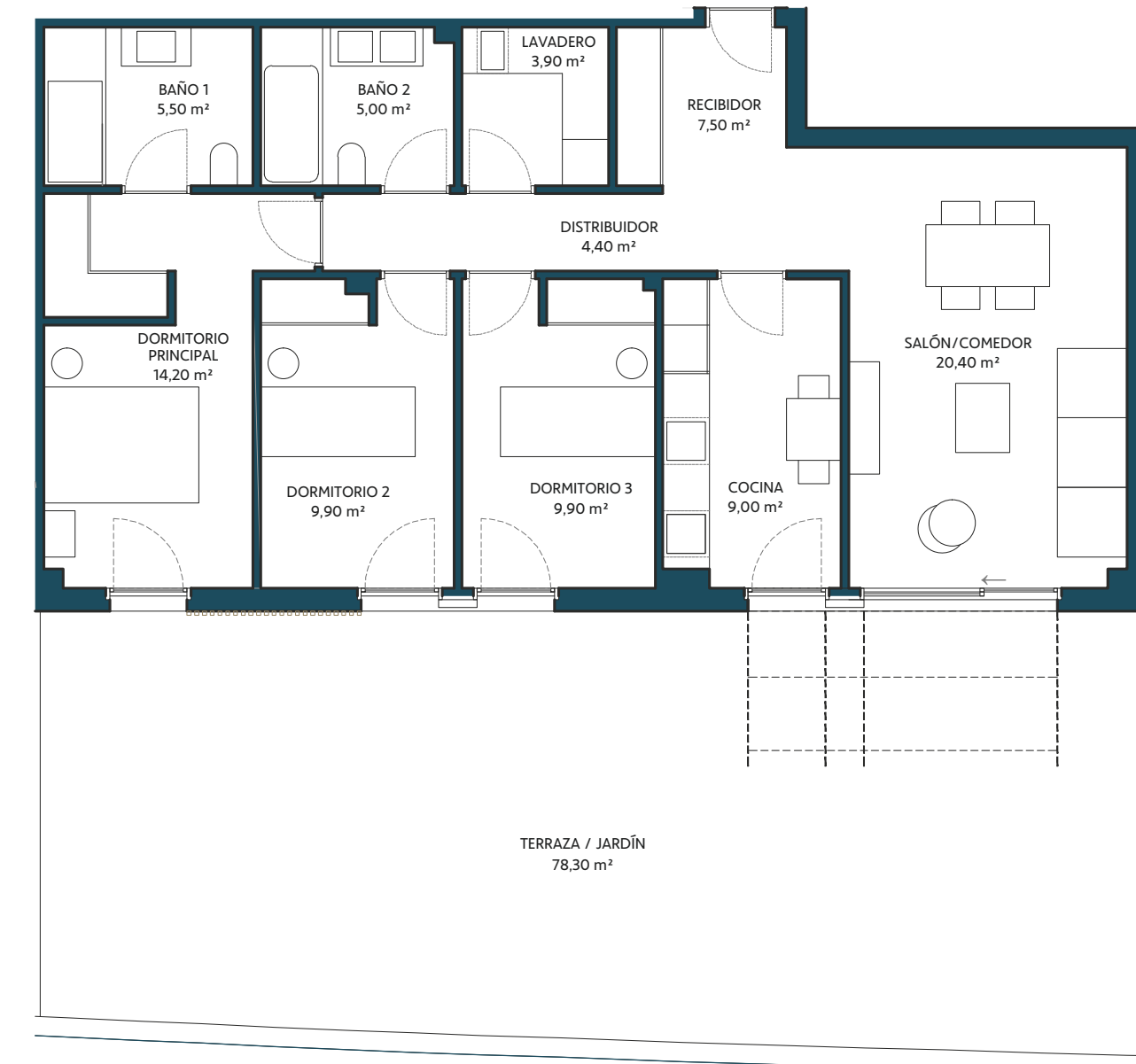
PLANTA BAJA CON ZONAS EXTERIORES
