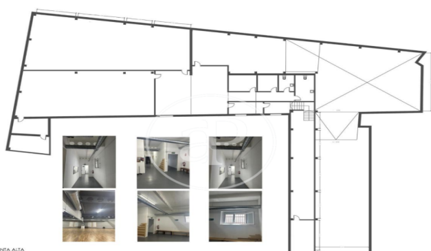
PLANTA ALTA ESTADO ACTUAL
