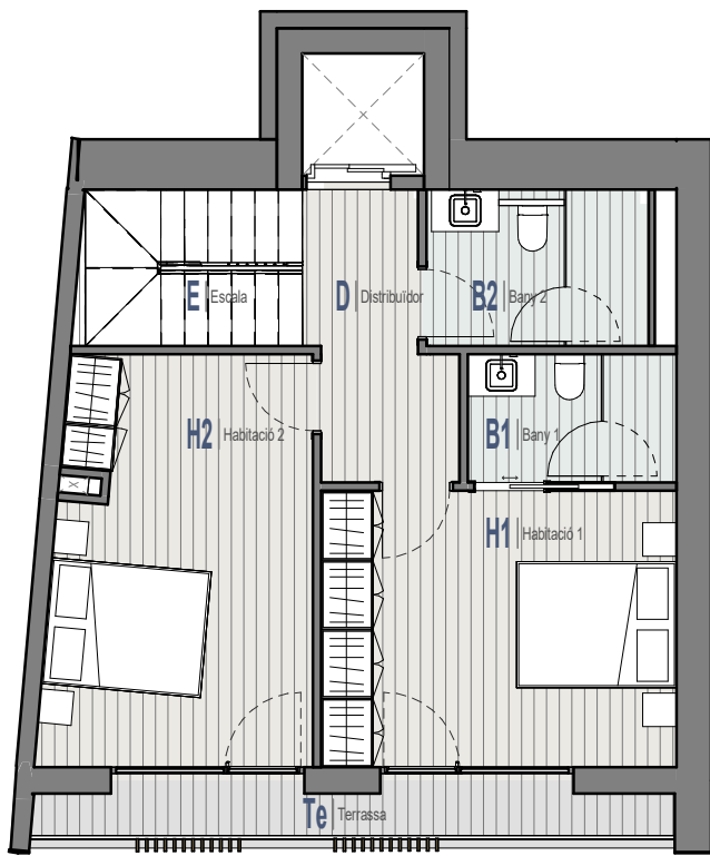
3 Planta Primera 1 : 100
