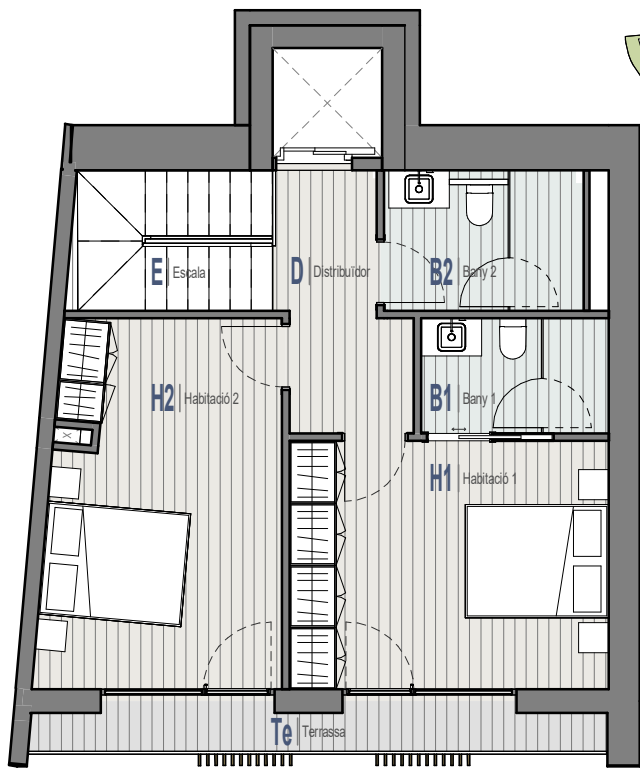
4 Planta Sotacoberta 1 : 100
