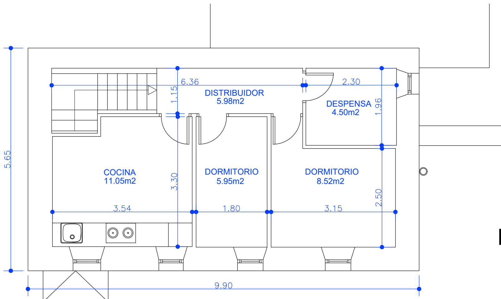
PLANTA PRIMERA
