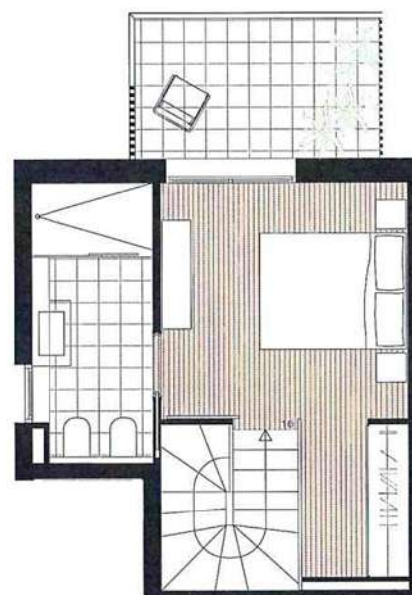
Planta Primera
