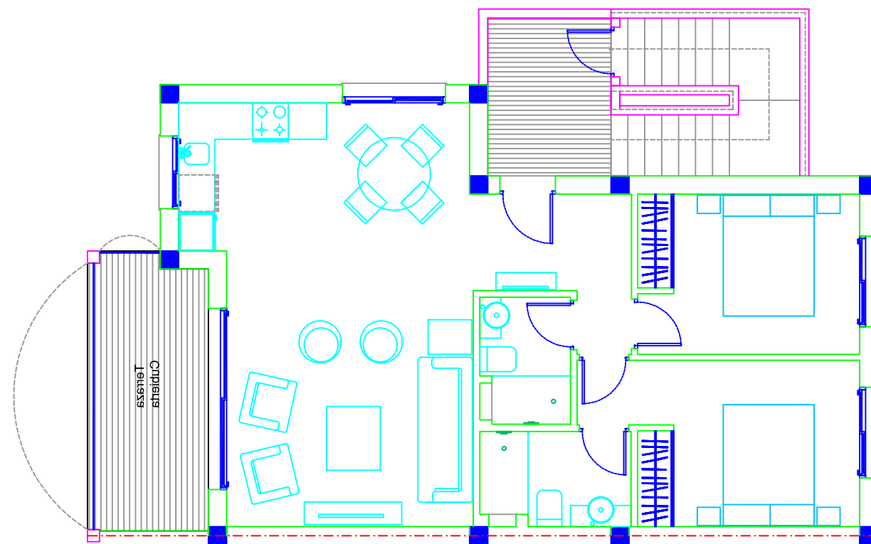
PLANTA PRIMERA
