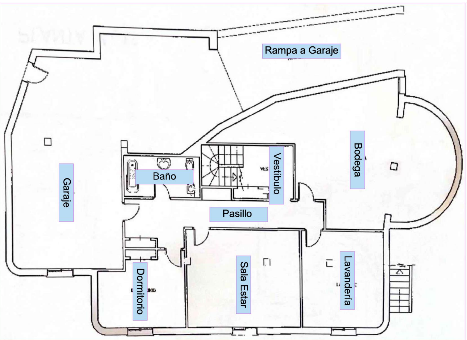
PLANTA BAJA VIVIENDA
