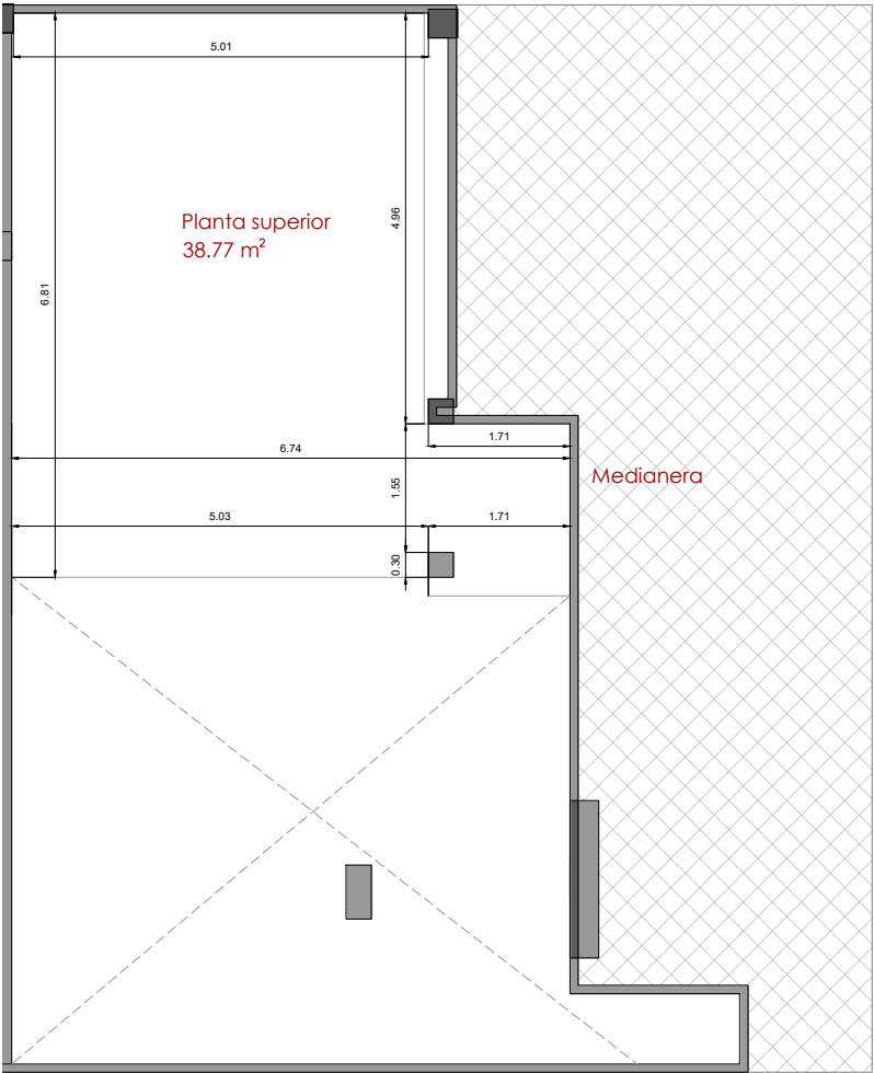
Planta superior
