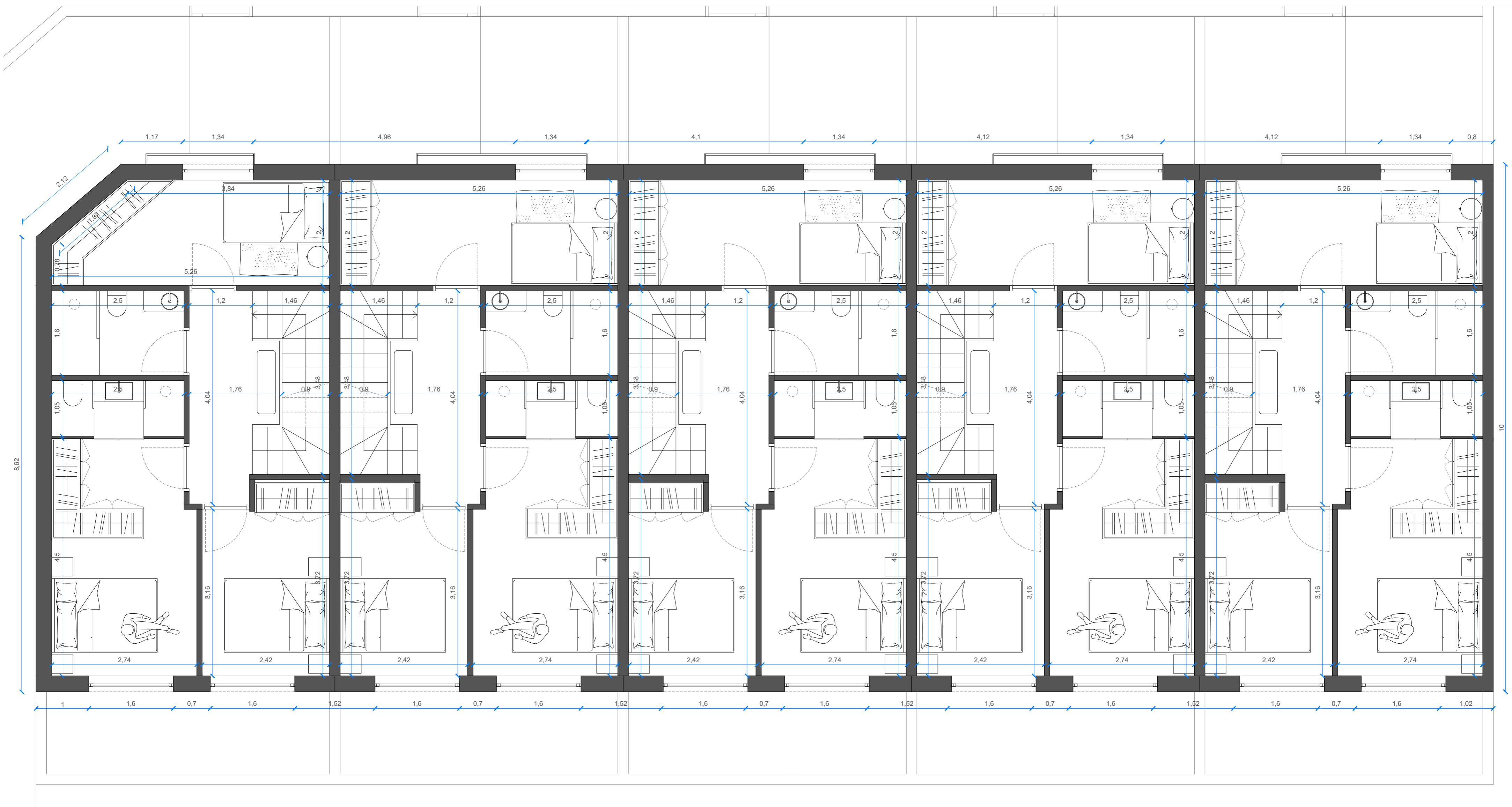
PLANTA PRIMERA
