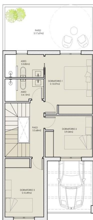
PLANTA ALTA S: 52,93m 2
