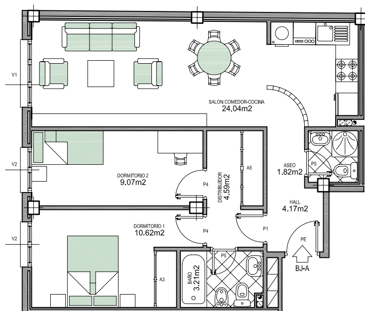
PLANTA BAJA CALLE TOLEDO 1A SUPERFICIE CONSTRUIDA BAJO A - 66.06 M2
