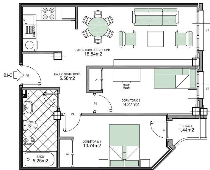
PLANTA BAJA CALLE TOLEDO 1A SUPERFICIE CONSTRUIDA BAJO C - 56.84 M2
