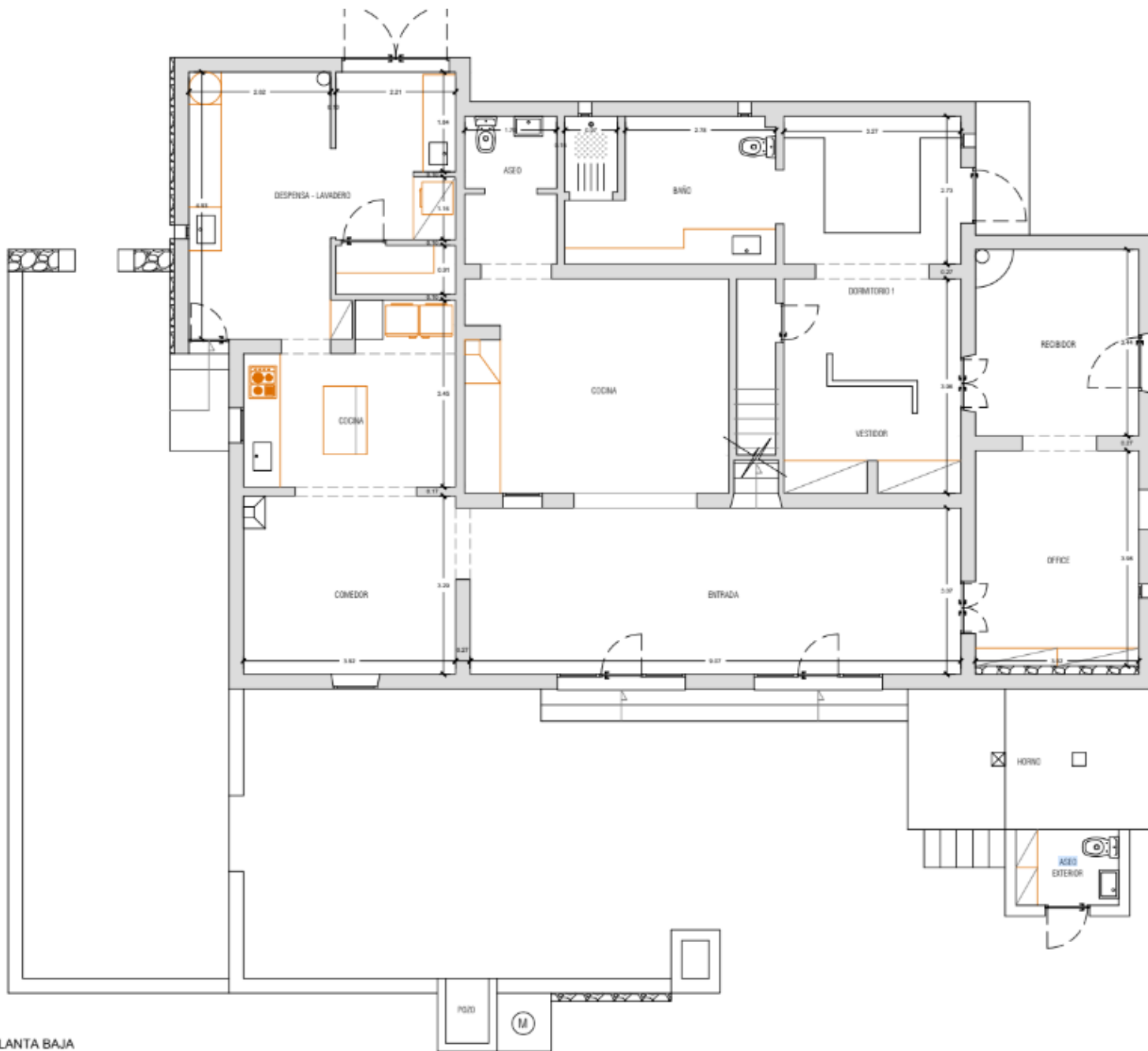
PLANTA BAJA Superficie construida 186.75m 2
