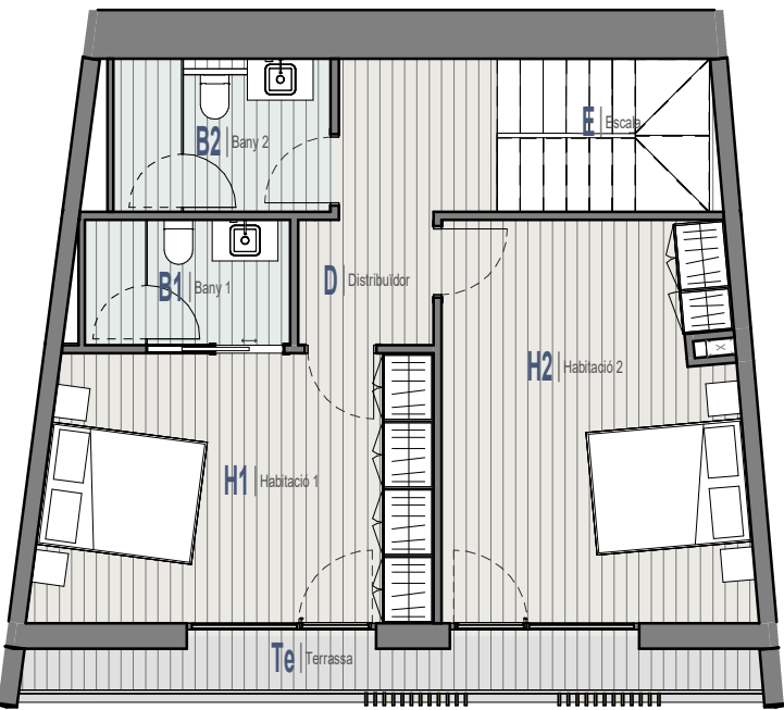
3 Planta Primera 1 : 100
