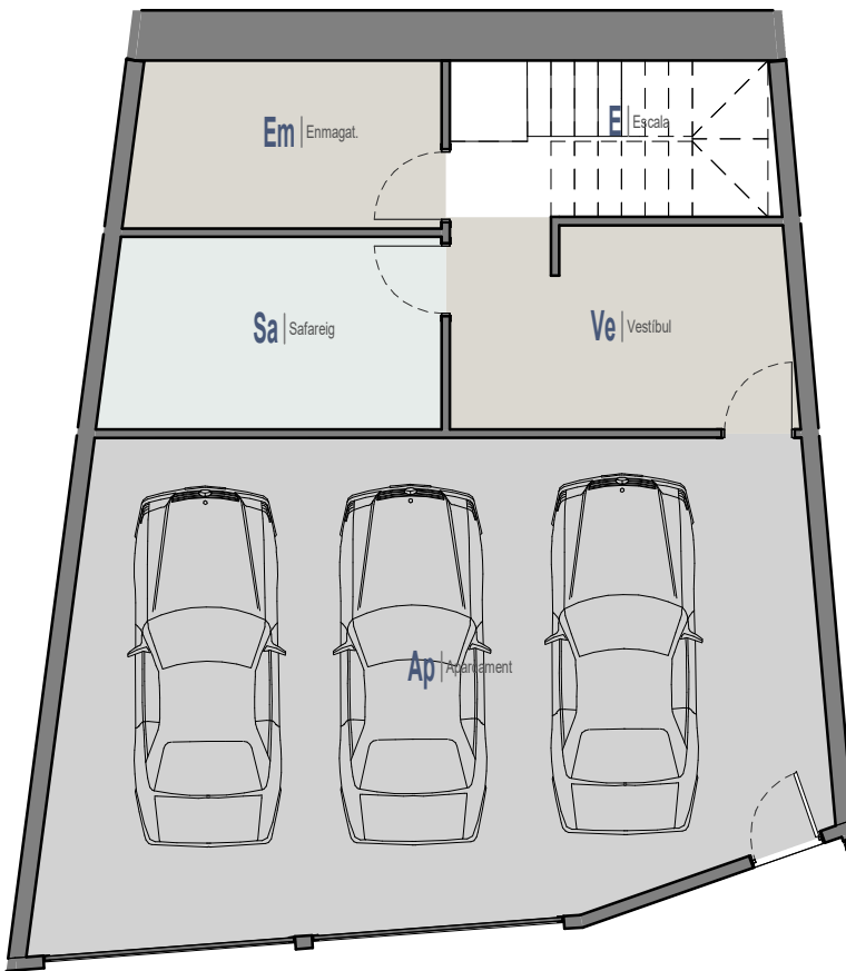
1 Planta Soterrani 1 : 100
