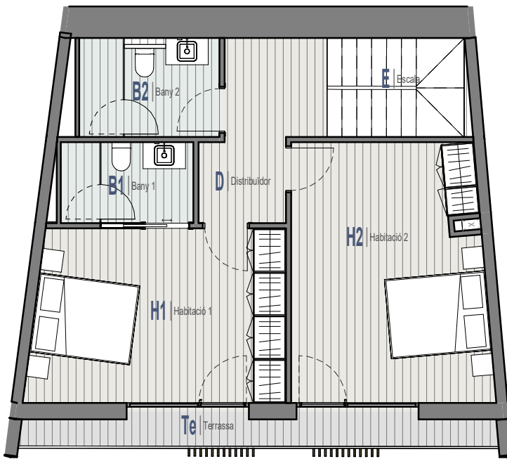
4 Planta Sotacoberta 1 : 100
