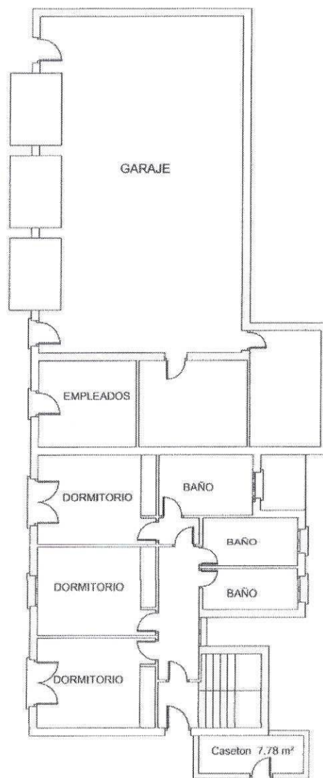
PLANTA BAJA
