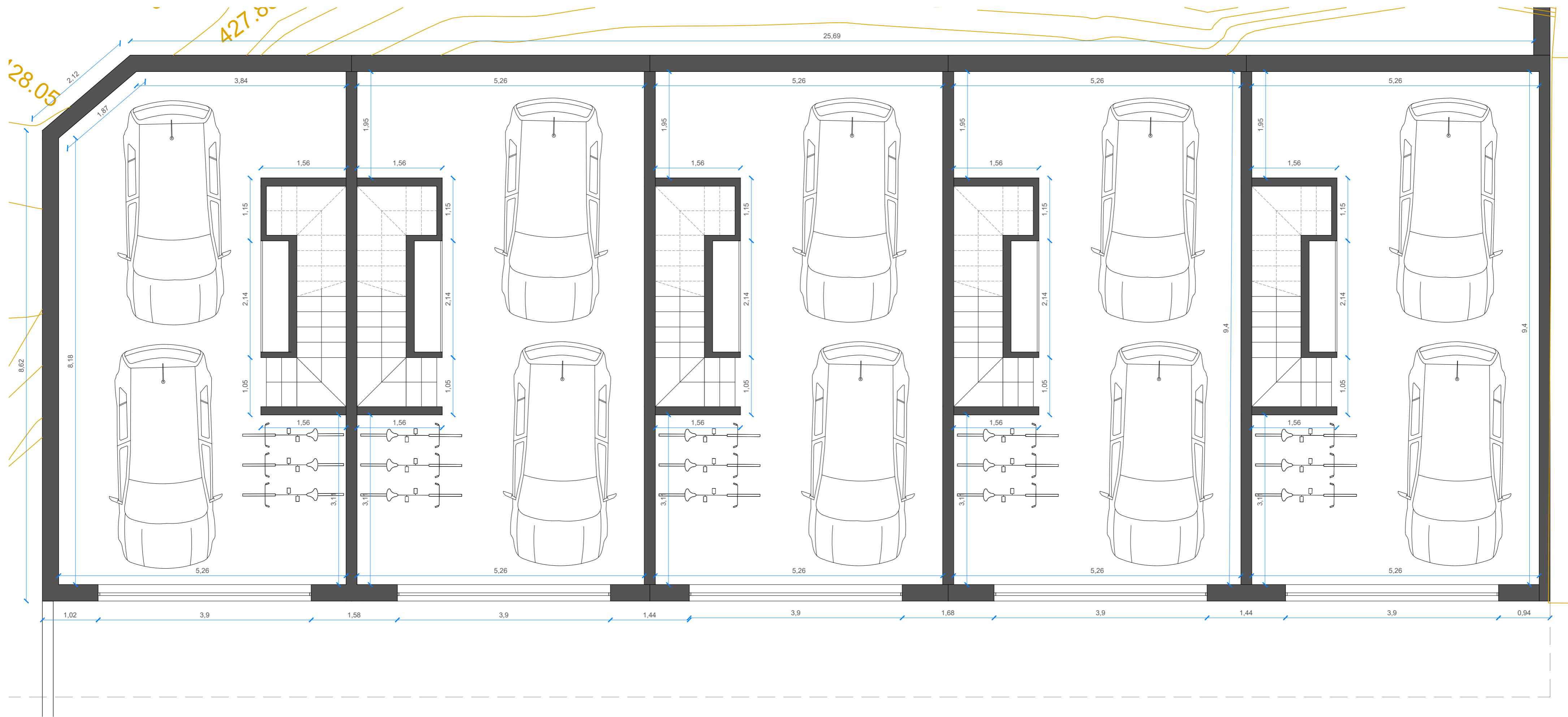
PLANTA SEMISOTERRANI
