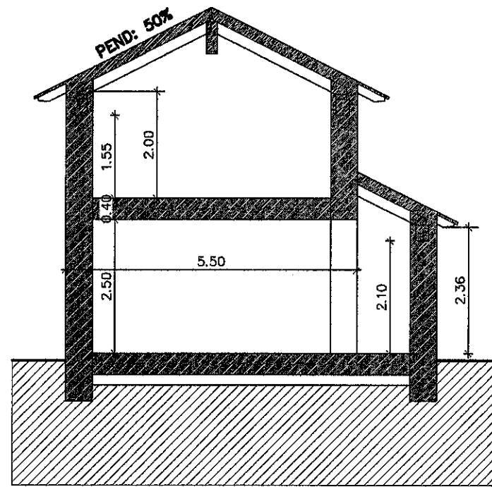
SECCION TRANSVERSAL A-A
