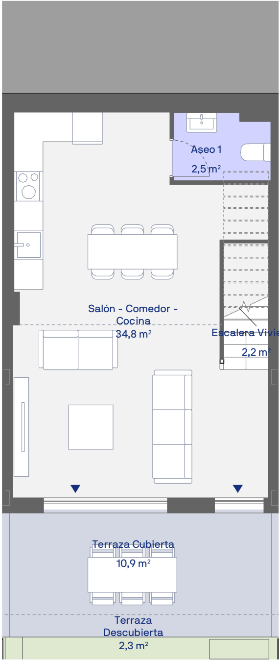
Planta baja
